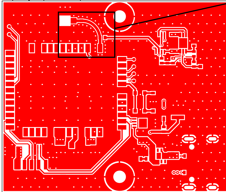
Top Layer (Scale 5:2)
